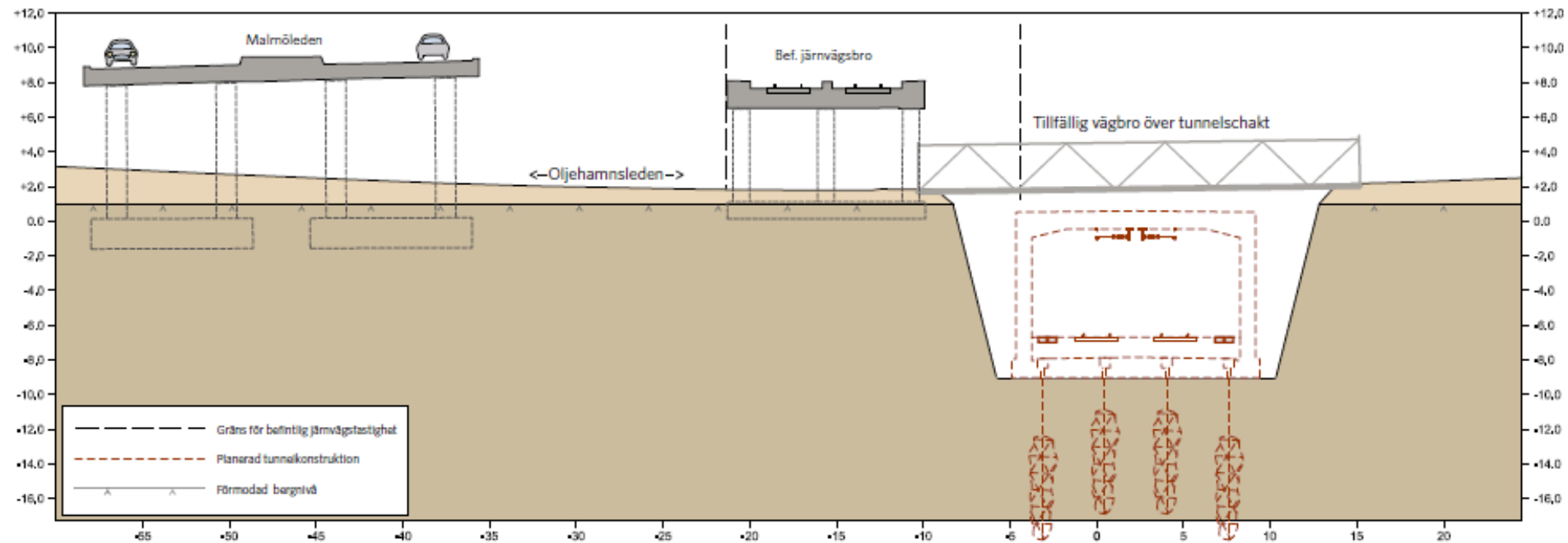
Tvärsektion km 244+840
